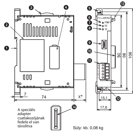
A méretek milliméterben vannak megadva. * FX3U-232-ADP: X = 7,5 mm, FX3U-485-ADP: X = 15,5 mm
