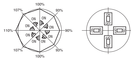
Fig.: Variación de la intensidad nominal si la orientación de montaje no es la vertical
