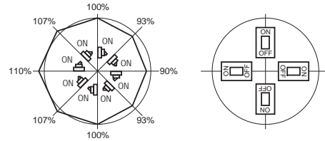
Ábra: A névleges áram változása függőlegestől eltérő beépítési helyzet esetén Tudnivaló: A termikus-elektromos vagy elektromos kioldású típusok kioldási karakterisztikája független a beépítési helyzettől.
