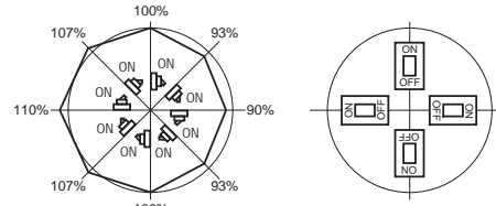
Рис.: Изменение номинального тока при отклонении монтажного положения от вертикали
