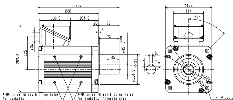
EM-AMFKT 7.5kW
