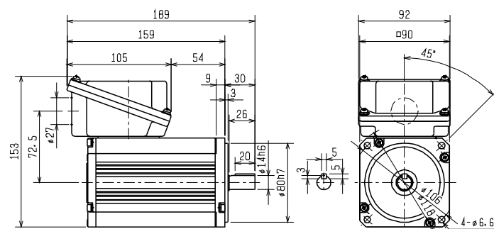
EM-AMFKT 0.75kW
