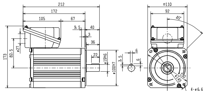
EM-AMFKT 0.4kW
