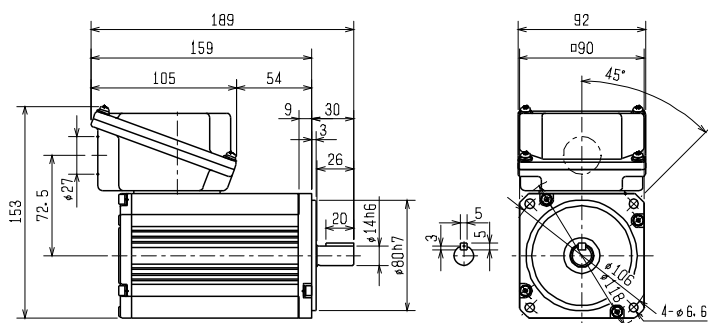
EM-AMFKT 0.4kW
